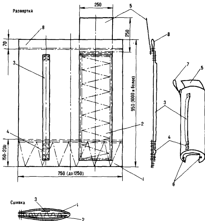
Рис. 233. Транспортный мешок
