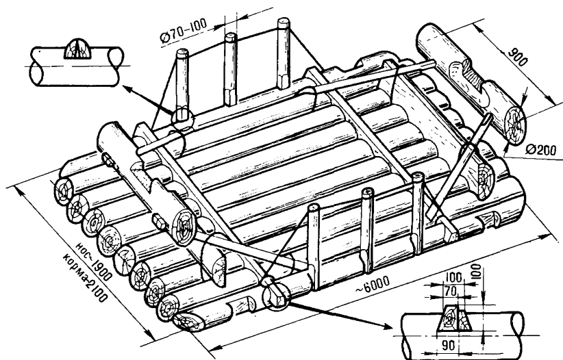
Рис. 139. Деревянный плот
