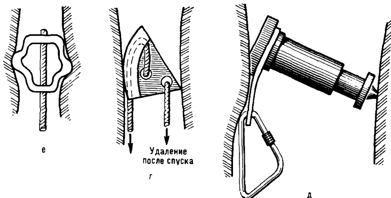
Рис.164 Варианты заклинивания закладных элементов различного типа :
