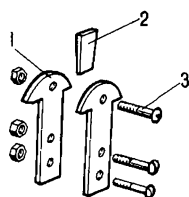
Рис.36. Крепление топора с помощью боковых накладок: 1-накладки;2-клин;3-болтики;4-темляк
