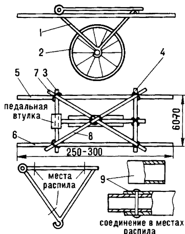
Рис. 40. Тележка на одном колесе (размеры в см)
