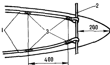
Рис.108. Пришивание обвязки:
