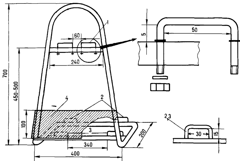
Рис. 12. Станок рюкзака:
