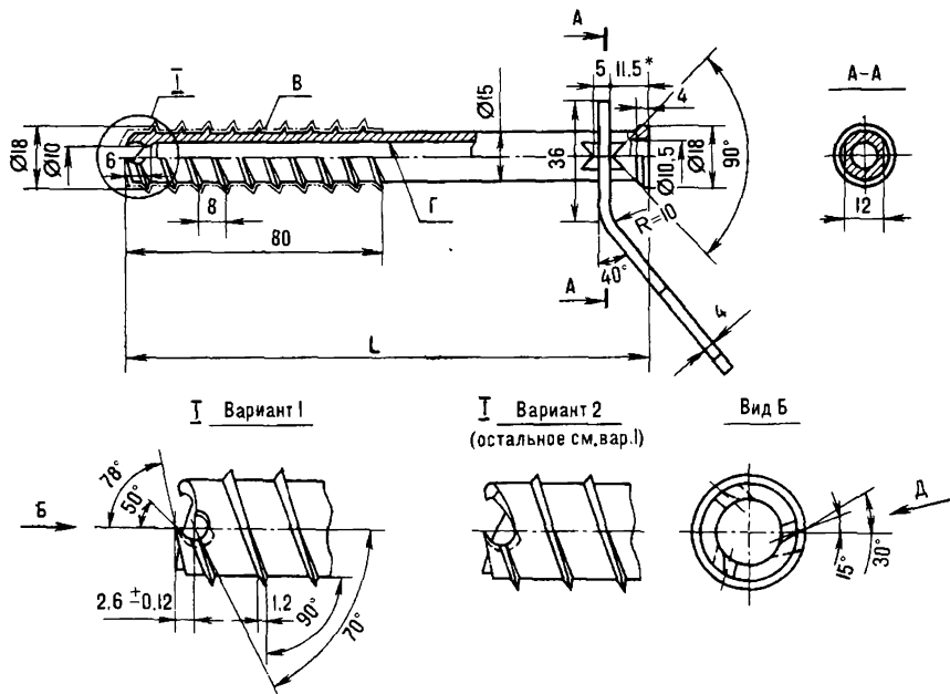
Рис. 167. Крюк-ледобур Твердость HRC 24...28. Серьгу обжечь, обеспечив зазор 0,5 мм. Острые кромки скруглить до R=0,5 мм, кроме резьбы и режущей коронки. Поверхность Г покрыть нитролаком. При изготовлении крюка из
