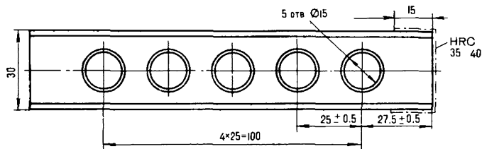
Рис 154. Швеллерные U-образные крючья:
