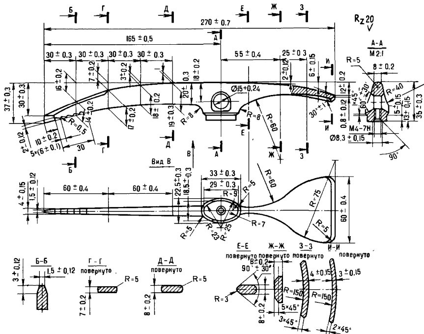
рис. 189 Головка ледоруба
