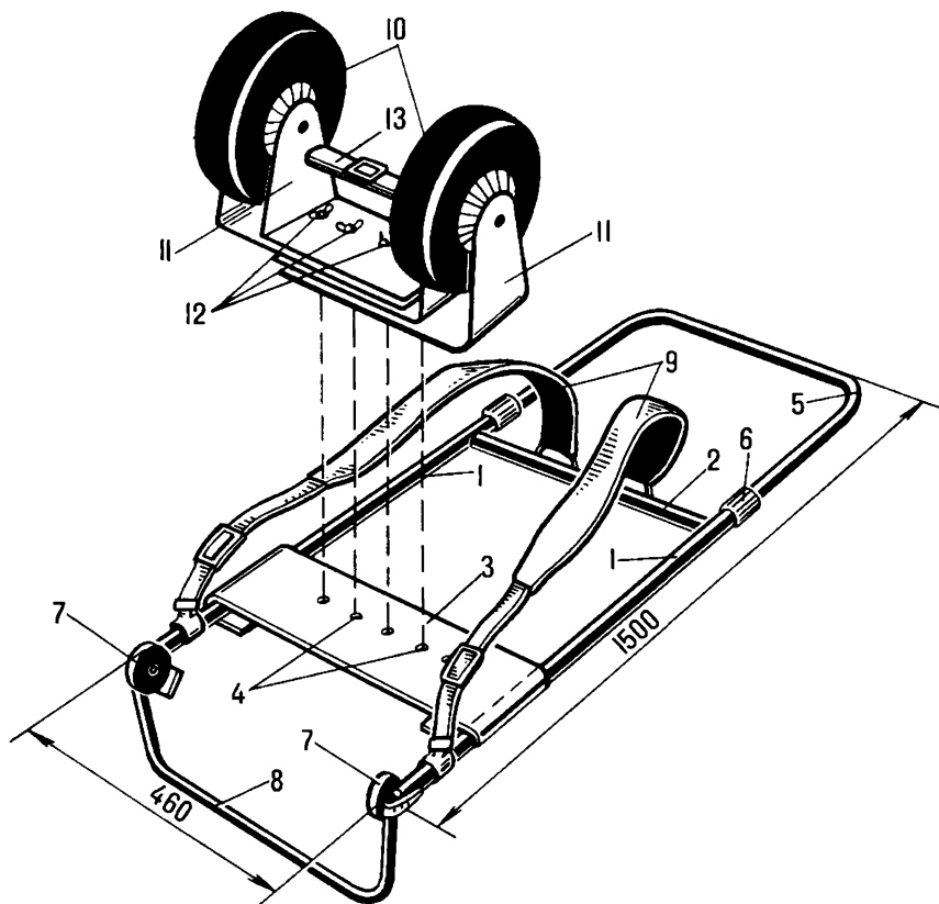
Рис. 41. Тележка со съёмными колесами
