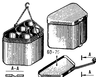
Рис.35.Комплект варочной посуды
