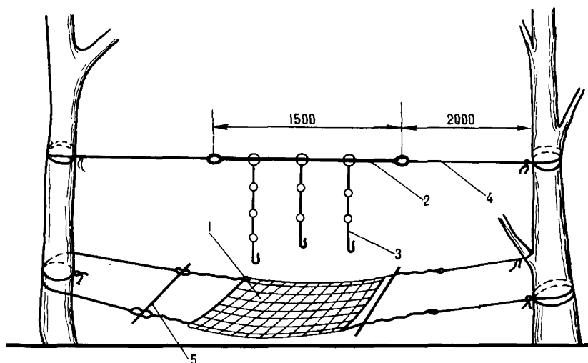
Рис. 56. Костровая сетка и тросик;
