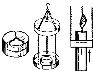
69. Палаточный светильник
