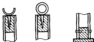
Рис. 6. Варианты окончания верхних и нижних концов трубок
