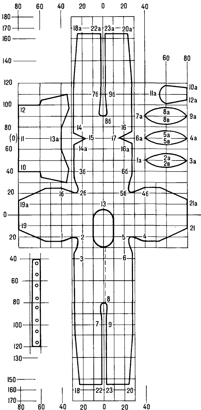
Рис. 211. Выкройка комбинезона (размеры в см)
