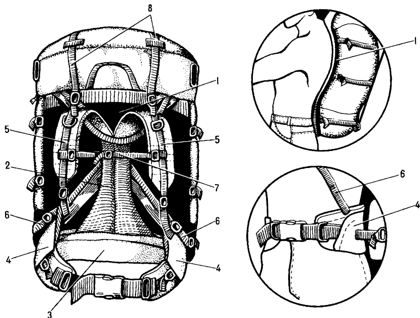
Рис. 14. Анатомический рюкзак:
