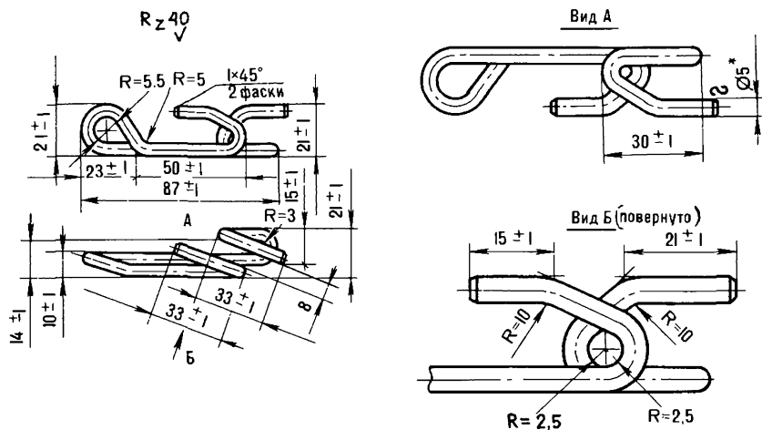
Рис. 202. Проволочный зажим
