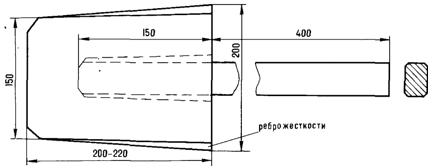
Рис. 77. Лавинная лопата
