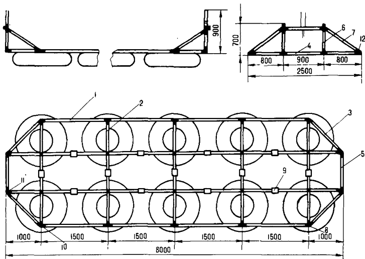
Рис 140. Плот с металлическим каркасом из модулей конструкции А Злобина, А Жукова, Д Сумбаева: 1—1,5 м (18 шт.), 2—1,2 м (10 шт.), 3—1,0 м (4 шт.), 4—0,9 м (2 шт.), 5—подгребница (2 шт.), 6—0,7 м (4 шт.), 7—1,4 м (4 шт.), 8—муфты (8 шт.), 9—муфты (13 шт.), 10—муфты (13 шт.), 11—муфты (4 шт.), 12—муфты для подгребниц (4 шт.) Вес труб—54 кг болтов и муфт—30 кг
