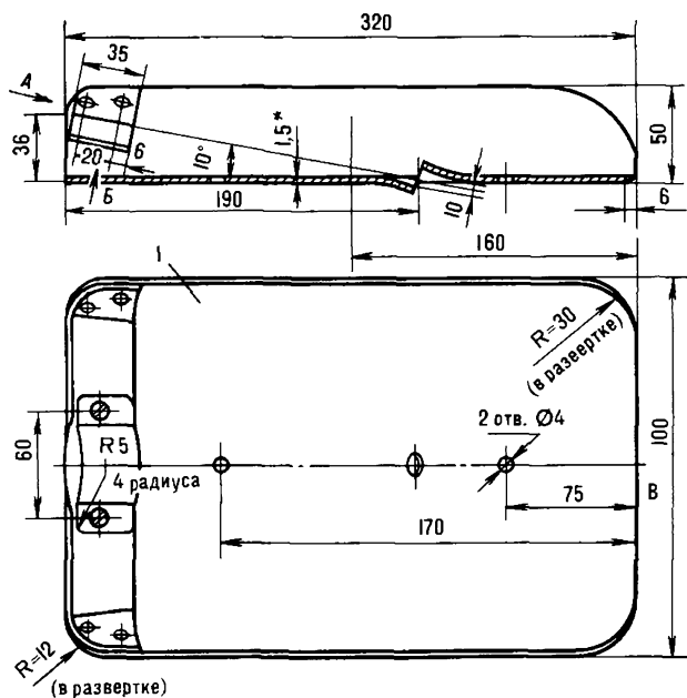
Рис.187.Снеговая лопата:
