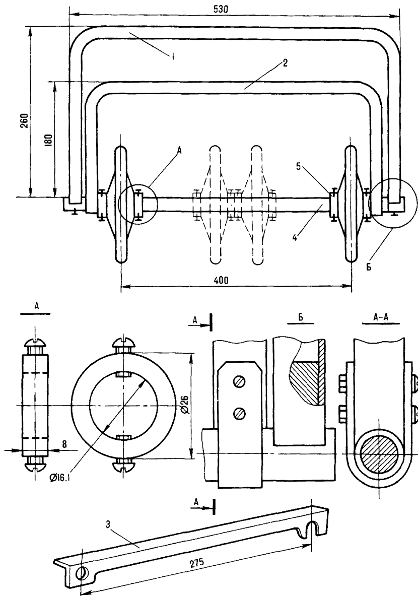
Рис. 39. Тележка-точка
