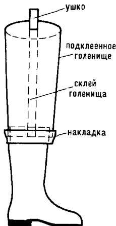
Рис. 28. Болотные сапоги
