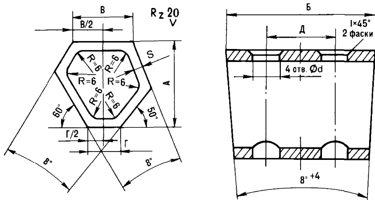
Рис.160.Гекса
