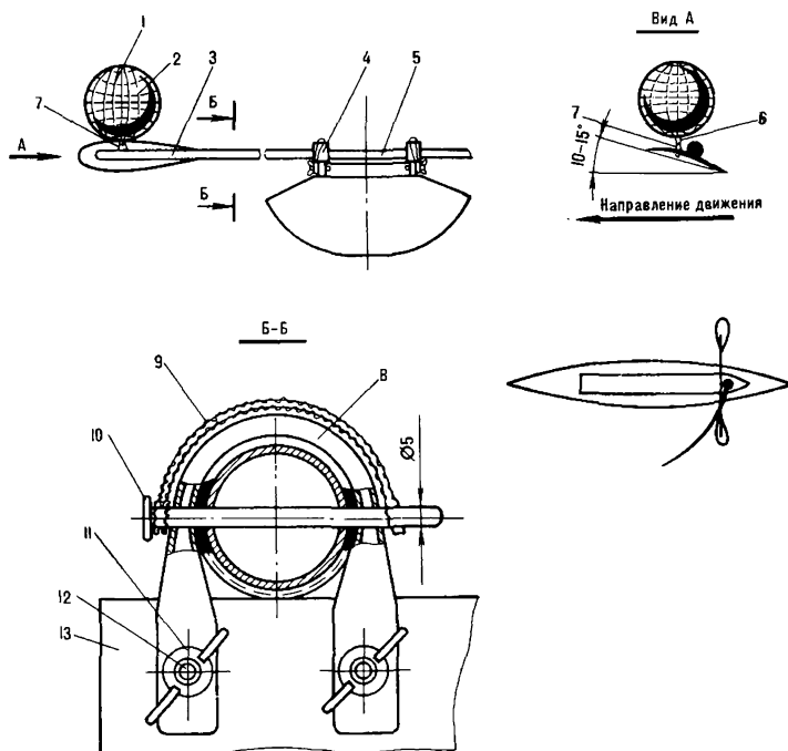
Рис. 149. Глиссирующее весло:
