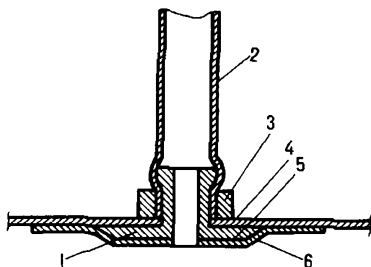
Рис.105. Вклейка штуцера:
