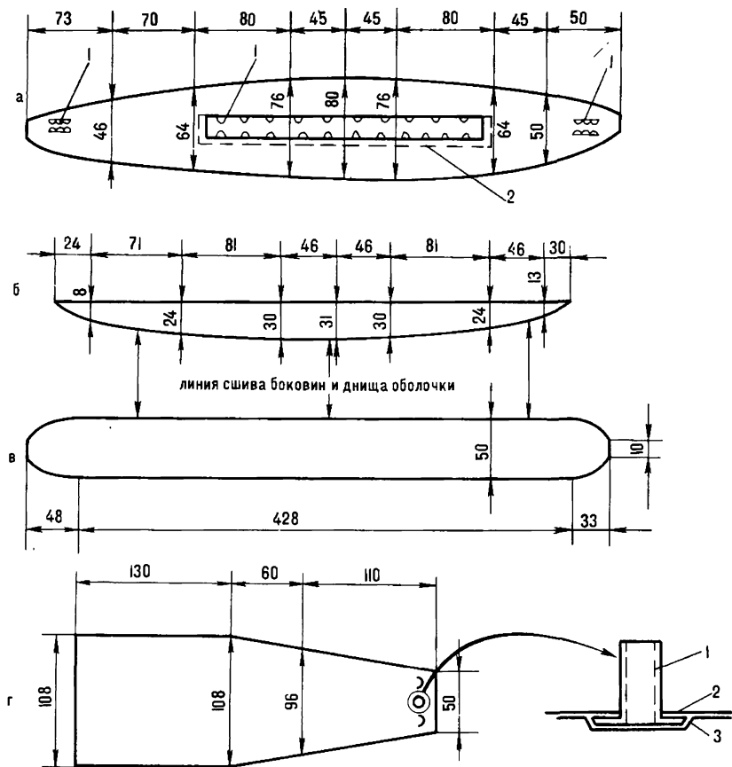
Рис.126.Выкройка оболочки и баллона (размеры в см):
