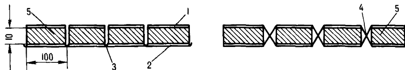
Рис. 10. Подстилочный коврик из пенопласта:
