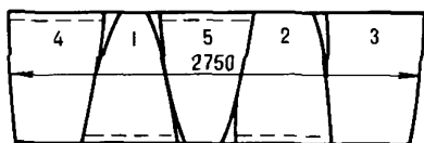
Рис.104. Вариант раскроя баллона
