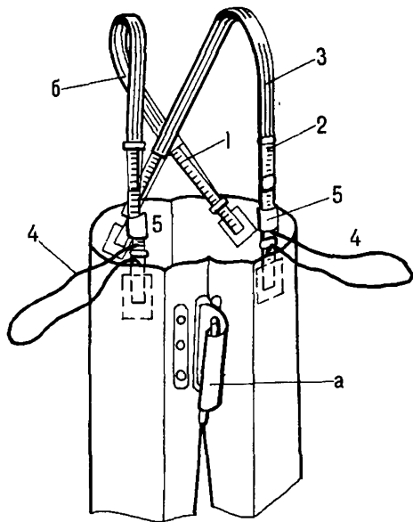
Рис. 212. Доработка брюк резинового гидрокостюма:
