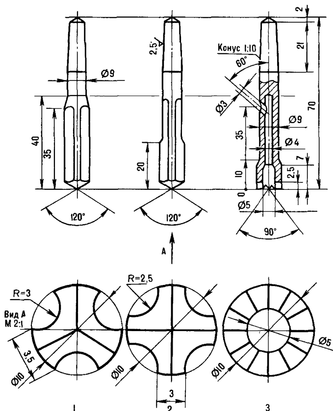
Рис. 231. Сменные бойки:
