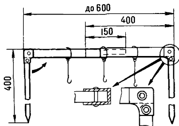
Рис. 31. Складная перекладина
