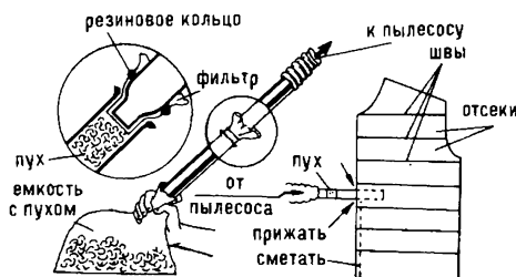
Рис. 26. Приспособление для наполнения куртки пухом
