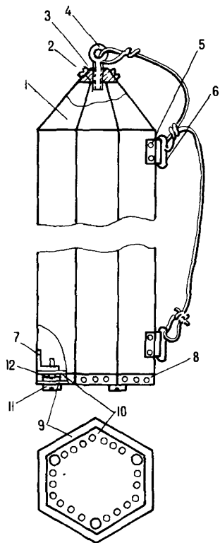
Рис. 234. Жесткий контейнер
