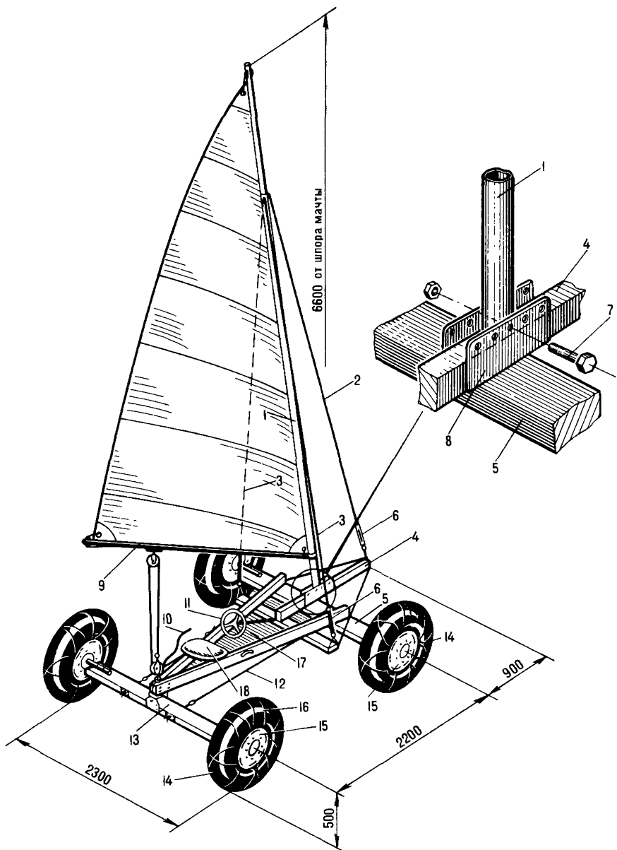
Рис. 79. Парусный снегокат
