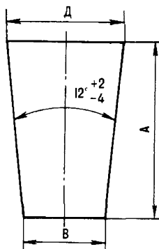
Рис. 159. Стоппер
