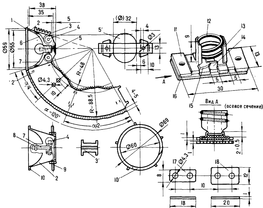
Рис. 222. Герметичный налобный фонарь
