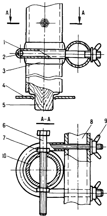
Рис.150. Пяртнерс на средней секции глизсирующего весла:
