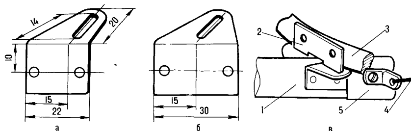
Рис.93.Кницы :
