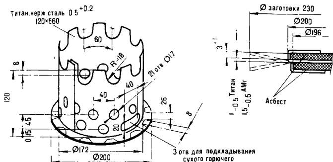
Рис 238. Гексагаз
