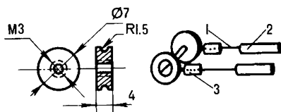
Рис.97. Крепление тросиков на штевнях: 1—тросик; 2—трубка ПХВ; 3—медная трубка с кернением
