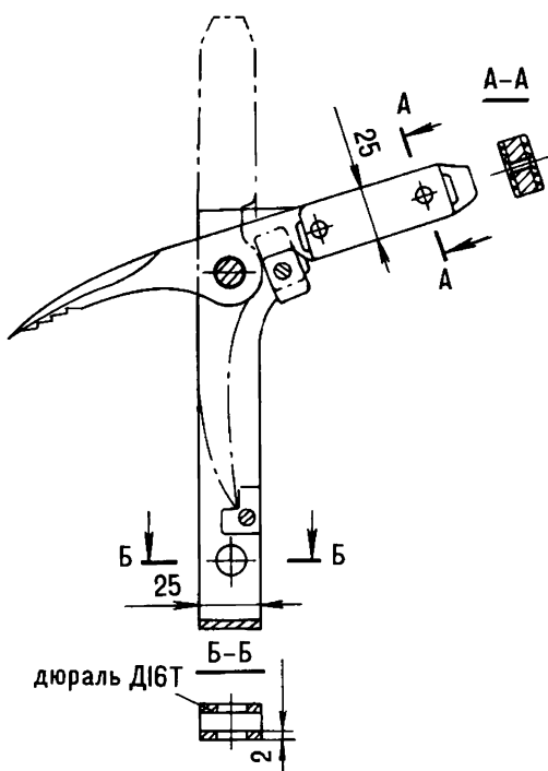
Рис. 170. Складывающийся якорный крюк
