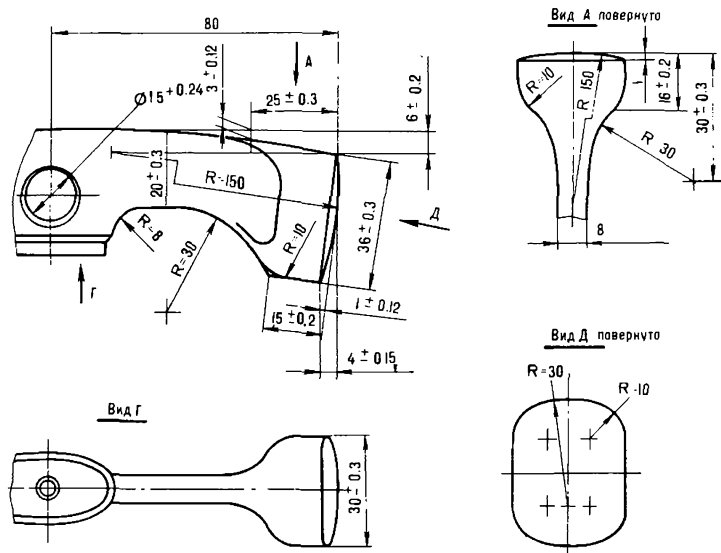
Рис.193.Боек айсбайля Конструкция и размеры коренной части головки даны под стандартный айсбайль (ОСТ 62-99-78) со сквозной стяжкой Боек (15-25 мм) каучук HCR 36 42. Покрытие Ц 9.хр.
