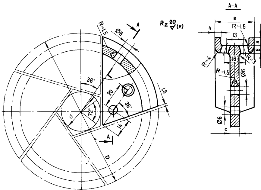
Рис.161.Самозаклинивающийся кулачок
