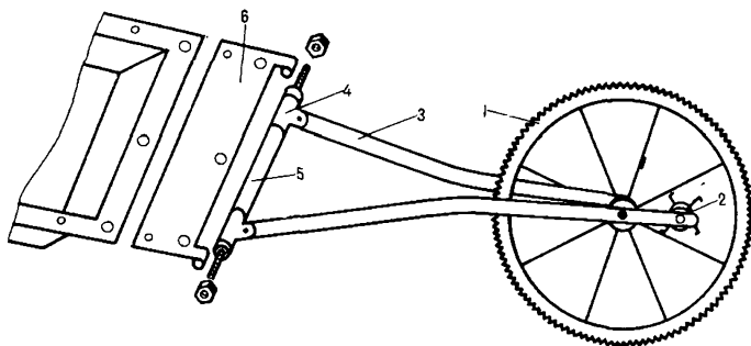
68. Одометр
