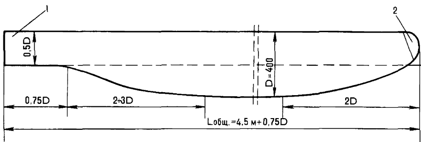
Рис.115, Основные размеры поплавка:
