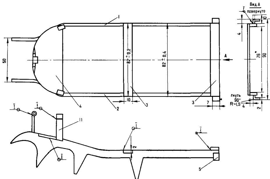
Рис. 179. Кошка конструкции Муравьева. Передок:
