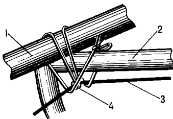
Рис.99. Натягивание силового тросика: 1—привальный брус; 2—шпангоут; 4— 3—тросик; 4—схватывающий узел
