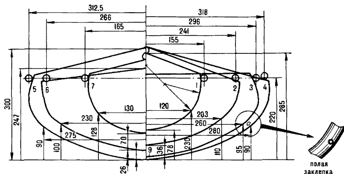
Рис. 86. Построение обводов шпангоутов
