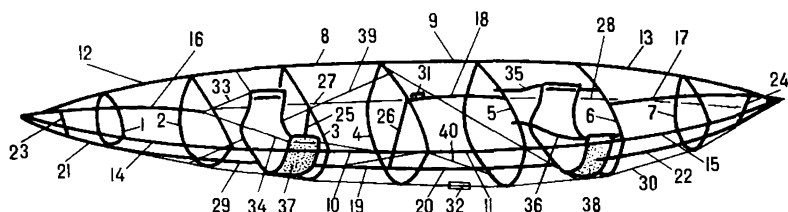
Рис. 85. Каркас КНБ-81:
