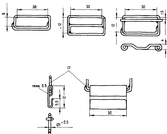
Рис. 215. Кольца, пряжки, петли, крючки
