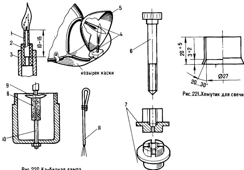
Рис. 220. Карбидная лампа
