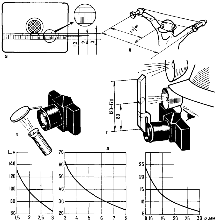
Рис. 237. Измерение расстояний "Зенитом"
