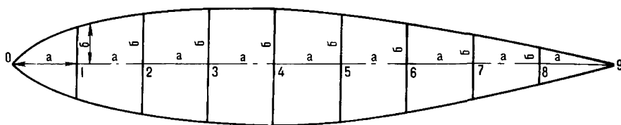
Рис.127.Раскрой баллона и оболочки
