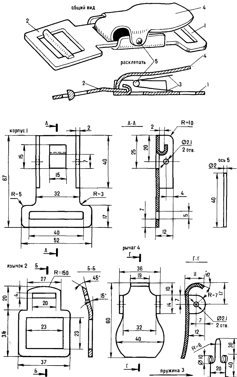
Рис. 18. Пряжка-самосброс
