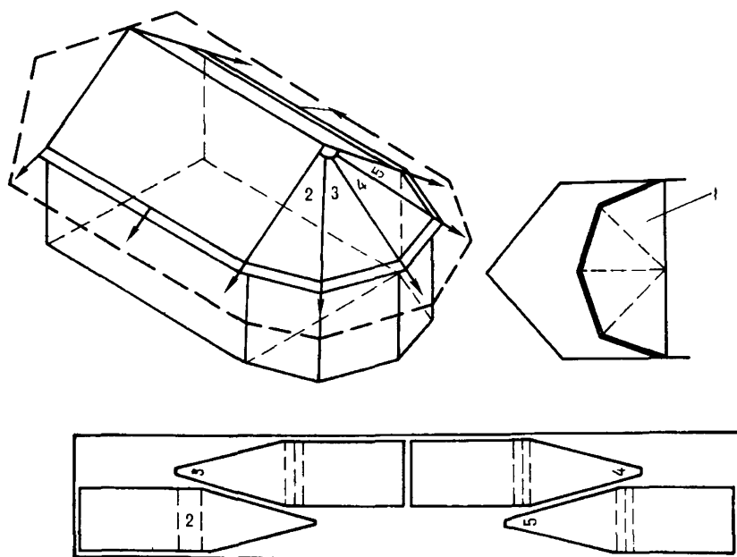
Рис. 4. Палатка с апсидой
