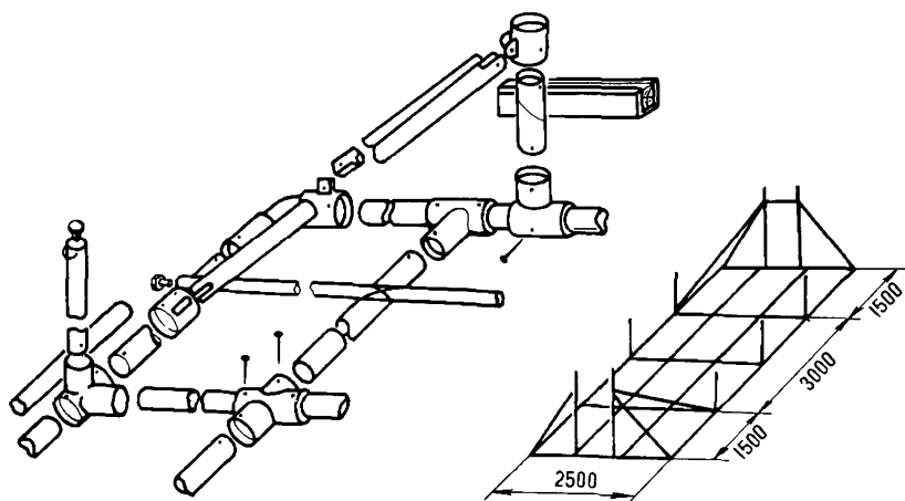
Рис. 135. Металлический каркас из труб с муфтовыми соединениями
