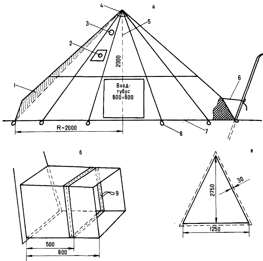
Рис. 42. Палатка "Чум" :
