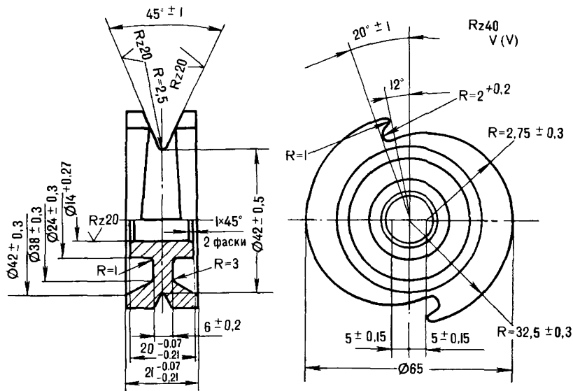
Рис. 204. Блок-тормоз. Шкив Неуказанные радиусы скруглений — 1 мм
