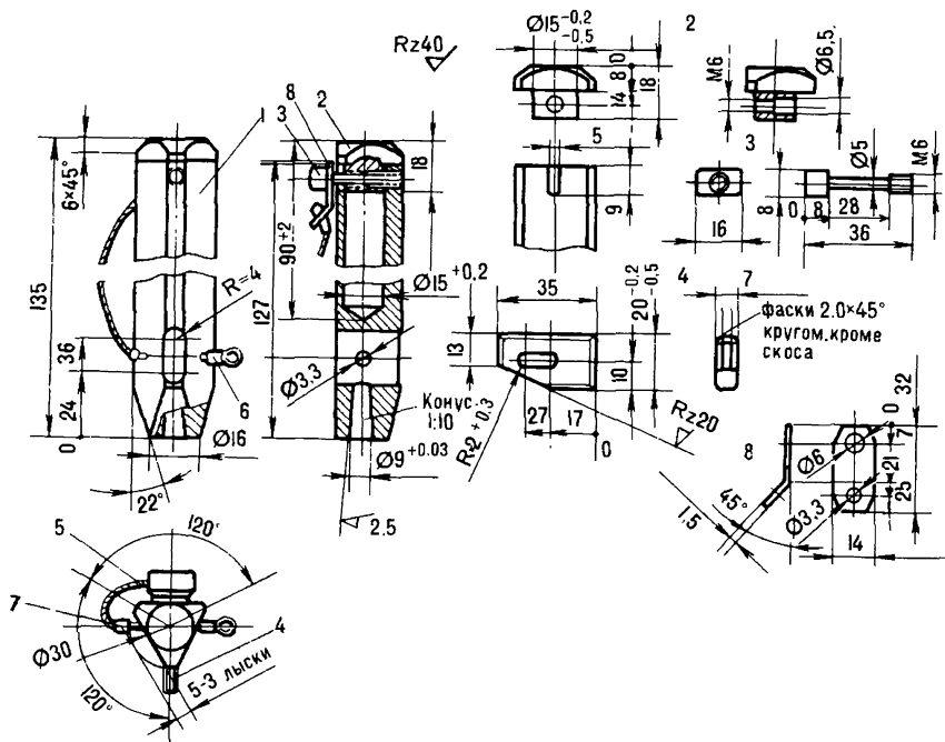
Рис. 230. Ручка шлямбура (дет. 1 и 2-Ст 45. НРС 40-45)
