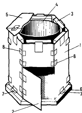
Рис. 53. Походная кухня
