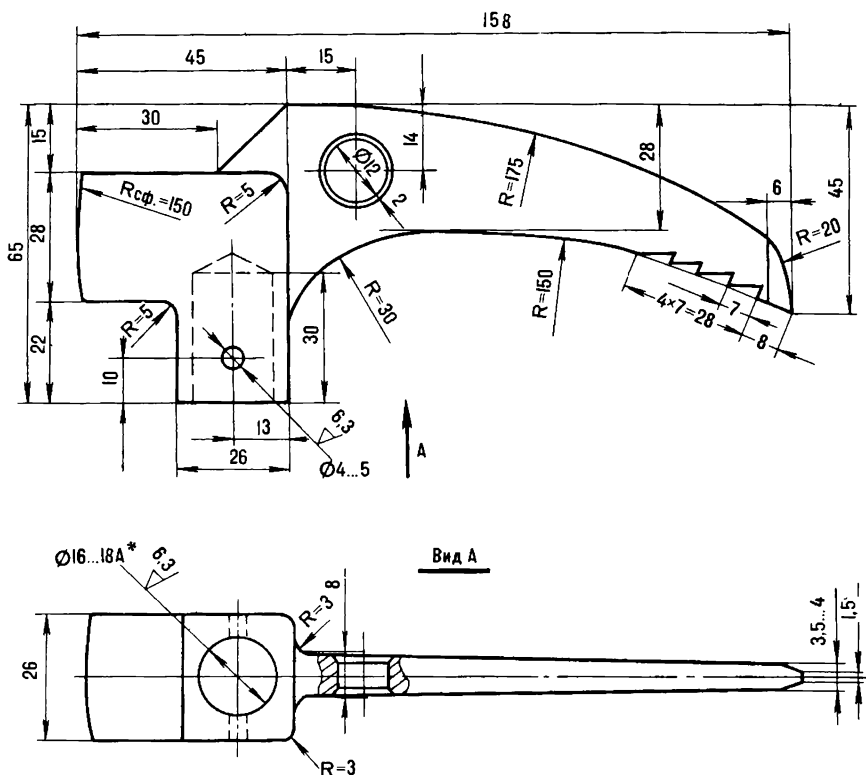
Рис. 171. Головка ледового молотка
