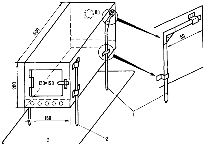
Рис. 49. Печка прямоугольная:
