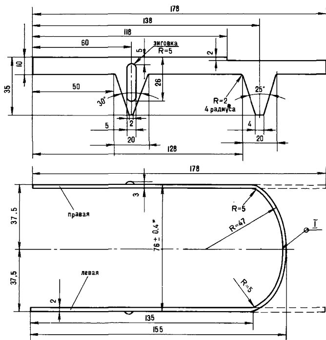
Рис.183 Кошка конструкции Муравьева. Боковины задника
