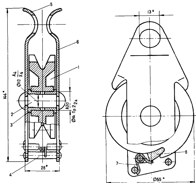
Рис. 203. Блок-тормоз
