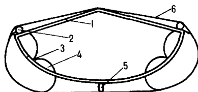
Рис. 84. Поперечный разрез КНБ-81: 1—шпангоут; 2—привальные бруссы; 3—опорные тросики; 4—баллоны; 5—кильсон; 6—оболочка
