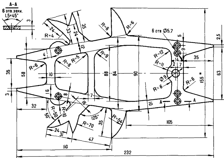
Рис. 176. Кошка 14-зубая, Передок (развертка) * - размер для справок
