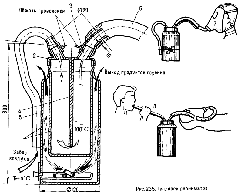
Рис. 235. Тепловой реаниматор
