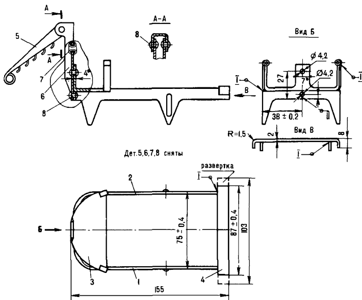
Рис. 180. Кошка конструкции Муравьева. Задник:
