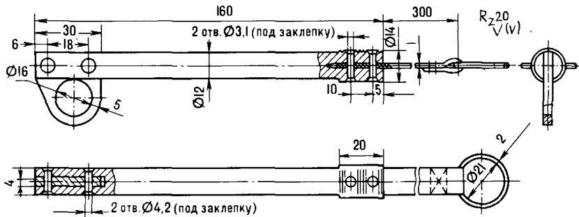
Рис. 173. Ледовый крюк-сбрасыватель
