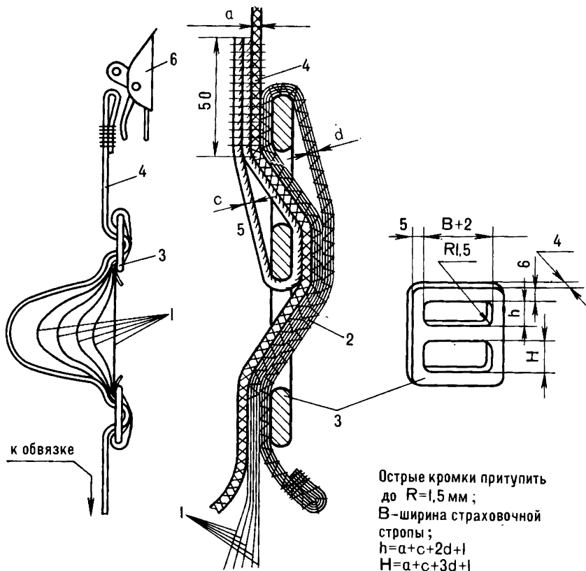
Рис.227. Пакетный ленточный амортизатор
