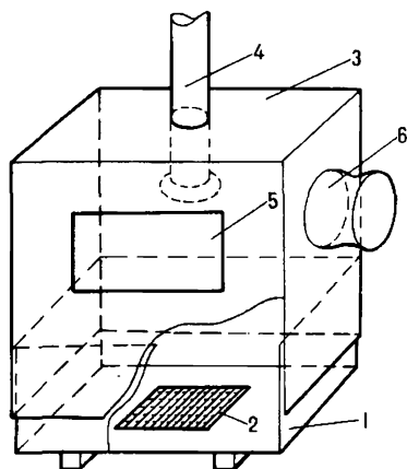
Рис. 25. Приспособление для отделения пуха
