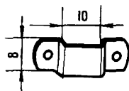
Рис. 89. Кница-скоба
