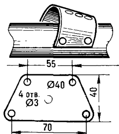
Рис.102. Стойка банки
