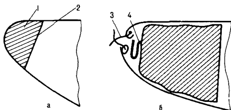
Рис. 119. Варианты оформления кормовой оконечности поплавков : а — глухая заделка кормы; б — заделка кормы с рукавом. 1 — половина резинового мячика диаметром 150–200 мм; 2 — линия склейки мячика с поплавком; 3 — стягивающий шнурок (штертик); 4 — скрученный и затянутый резиновым бинтом кормовой рукав
