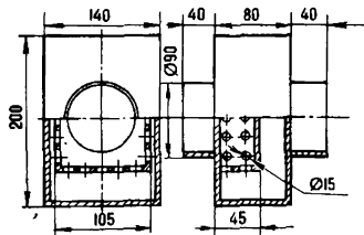
Рис. 55. Искрогаситель-экономайзер
