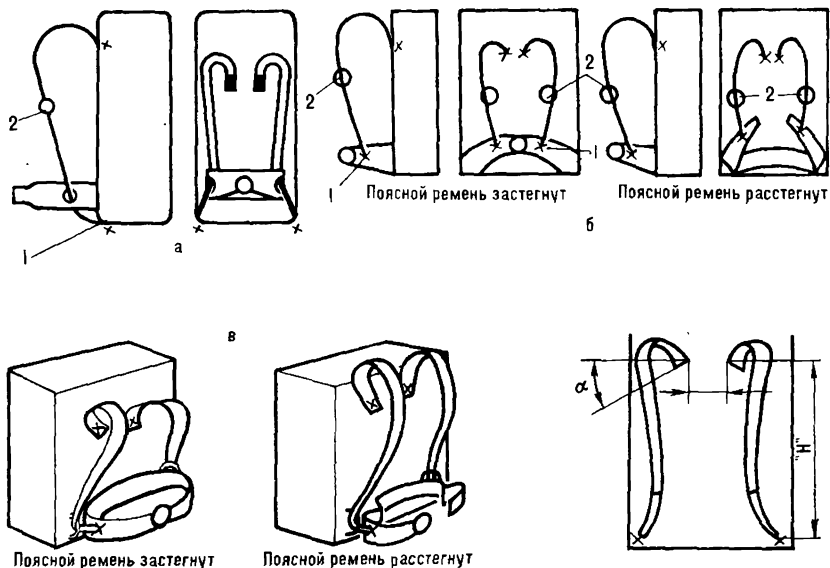
Рис. 16. Варианты крепления плечевых ремней;
