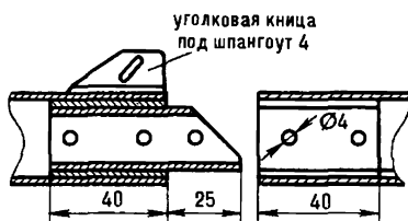
Рис. 92. Стыковка кильсона
