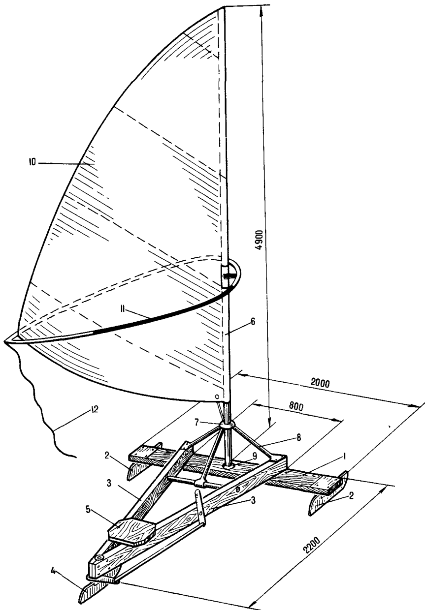
Рис. 78. Коньковый буер
