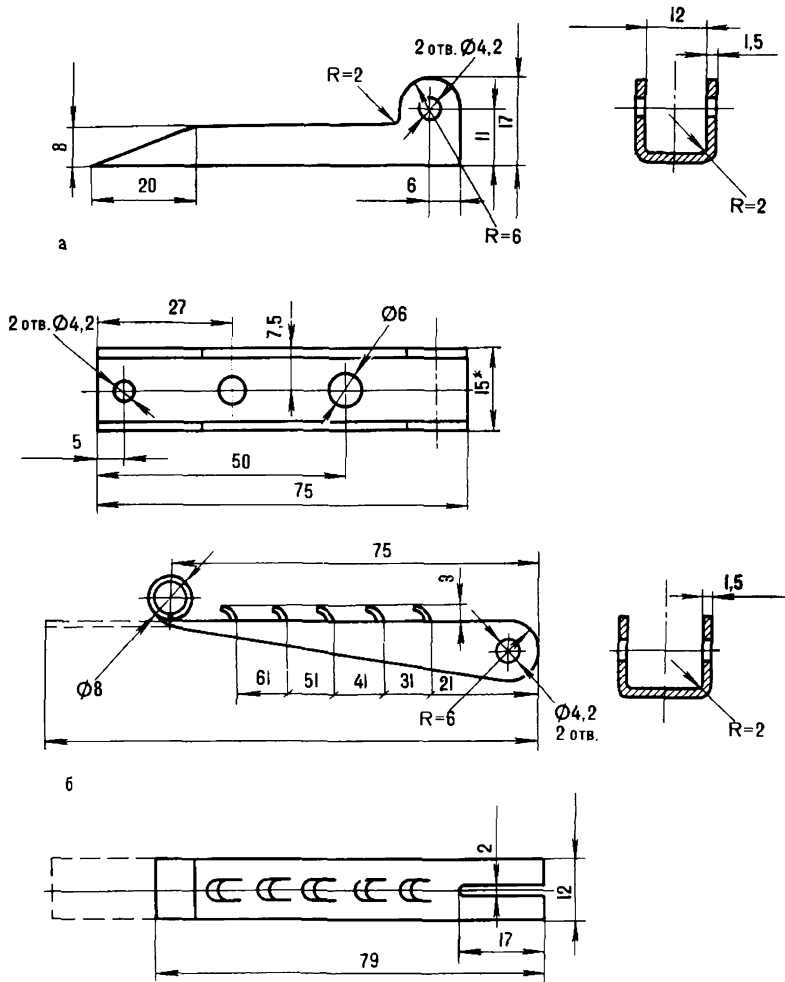
Рис.184. Кошка конструкции Муравьева: стойка (а) и замок (б) Острые кромки притупить. Материал: сталь Х18. шероховатость поверхности R_z 40 . * — размер для справки
