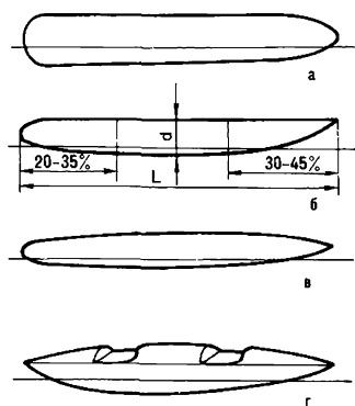
Рис. 112. Форма надувных поплавков: а — цилиндрическая; б — промежуточная; в — веретенообразная; г — верблюж
