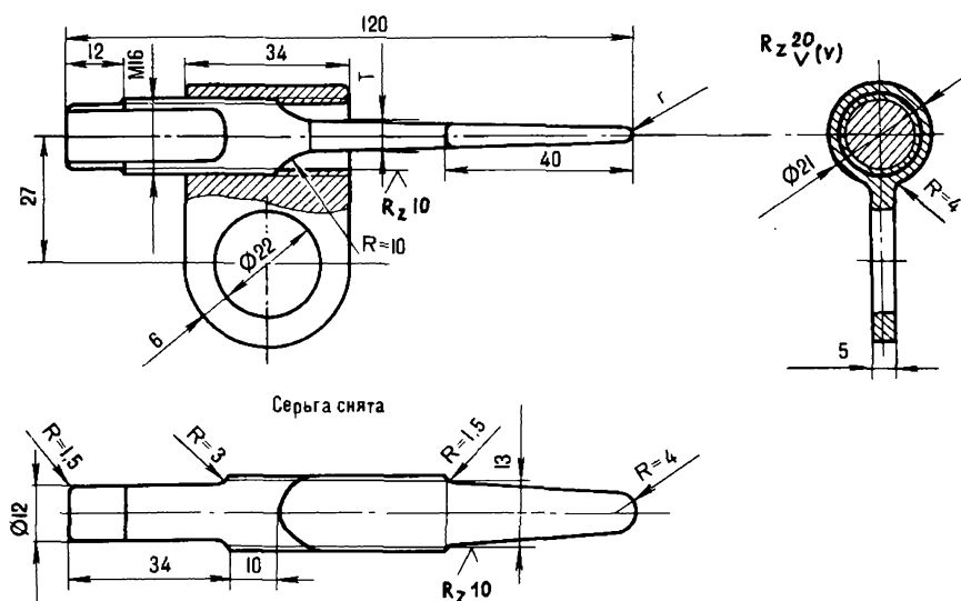
Рис.156. Крюк-винт
