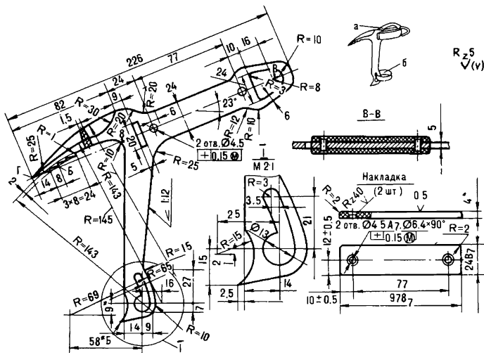
Рис. 169. Якорный крюк (накладки сняты)
