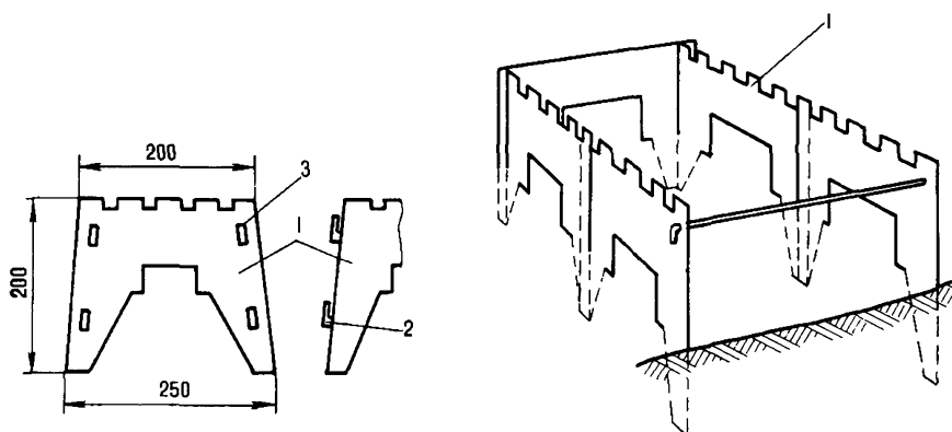
Рис.33. Таганок из фигурных пластин
