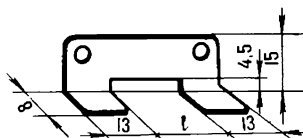
Рис.96.Лапчатая кница
