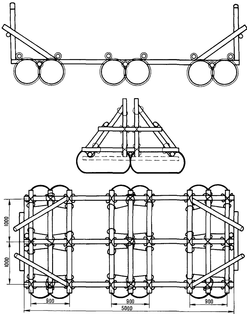
Рис. 141. Плот с поперечно расположенными поплавками конструкции А. Чернышева
