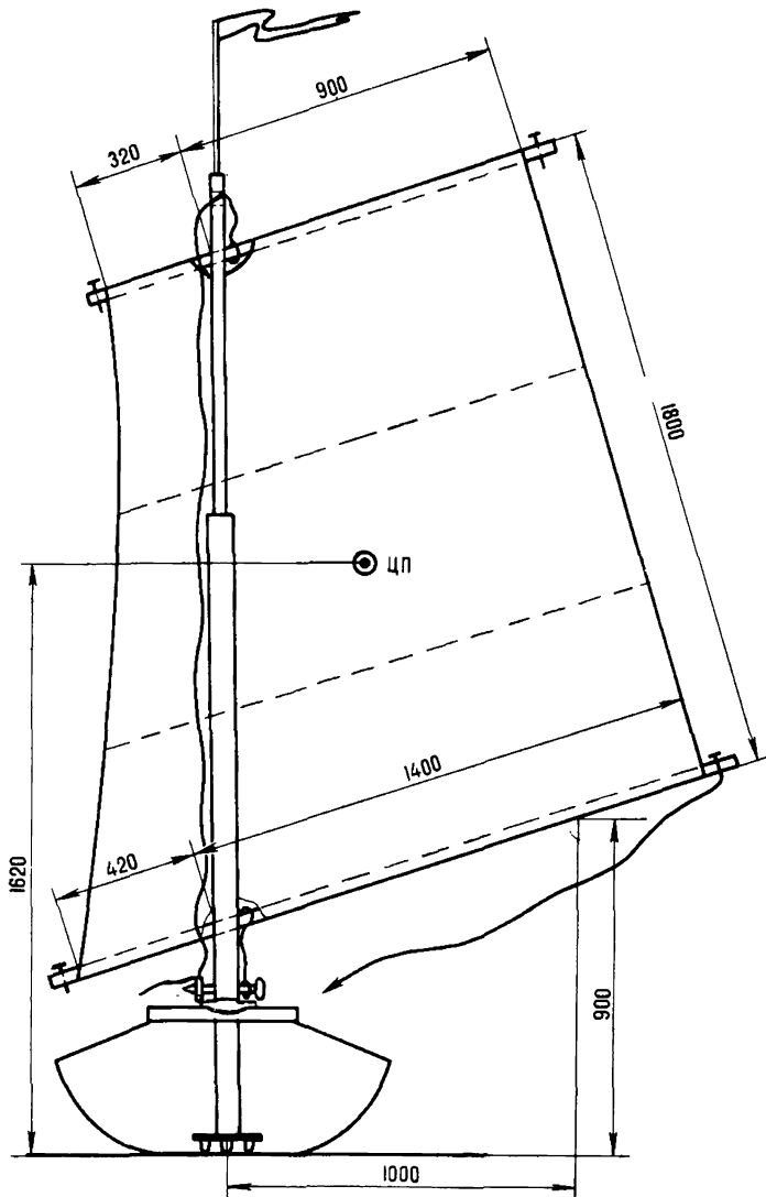
Рис.146.Усовершенствованный рейковый парус (площадь—2,85 м)
