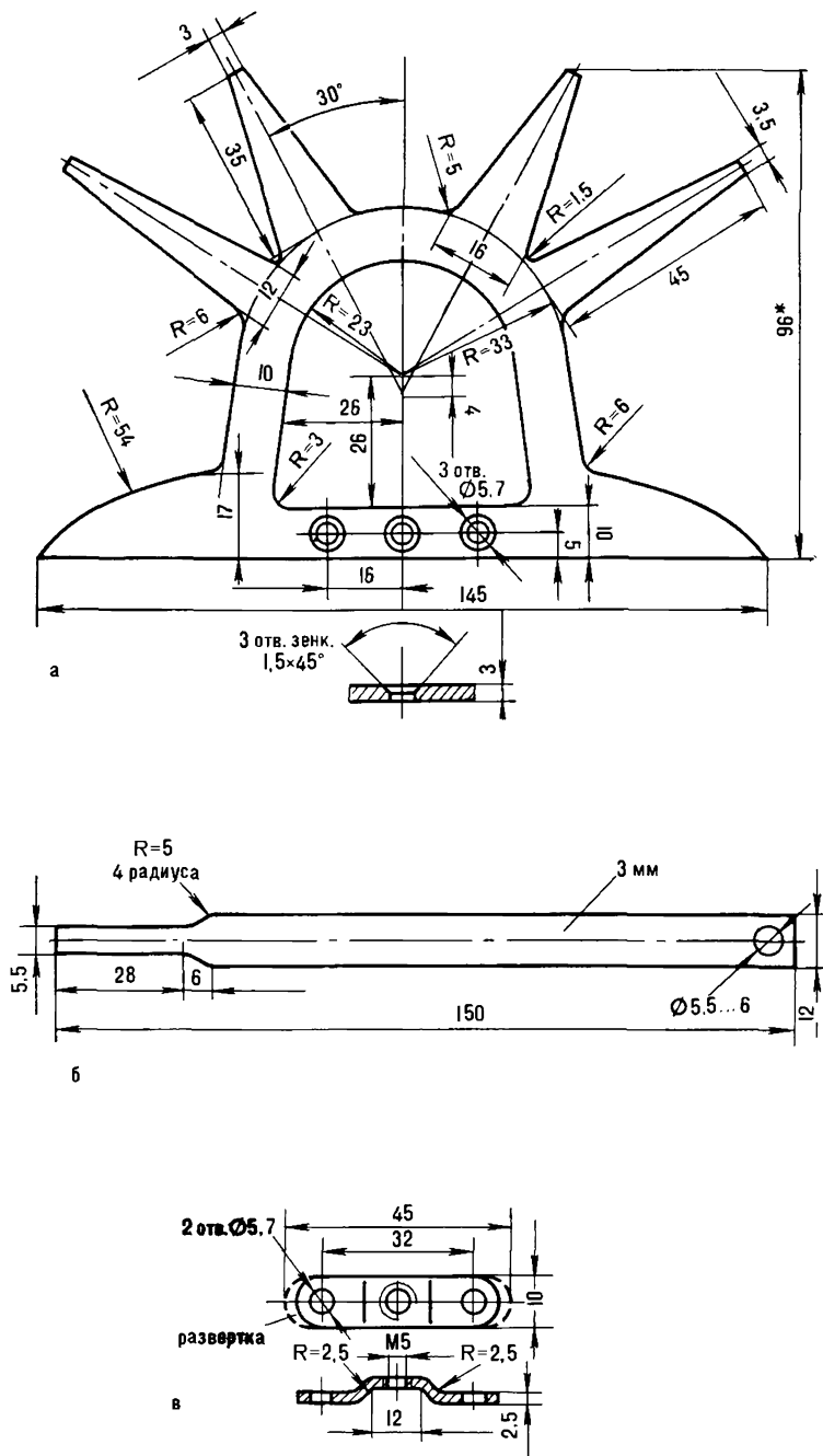
Рис.177.Кошка 14-зубая.Задник (развертка);
