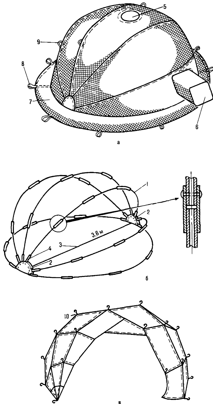
Рис. 47. Двухслойная каркасная палатка: а-общий вид; б-каркас; в-внутренний слой, 1-трубки каркаса; 2-"звездочки"; 3-тросик; 4-патрубки; 5-вентиляционный тубус; 6-вход-тубус; 7-"юбка"; 8-ниж- ние петли; 9-петли для оттяжек; 10-крючки для подвески внутреннего слоя
