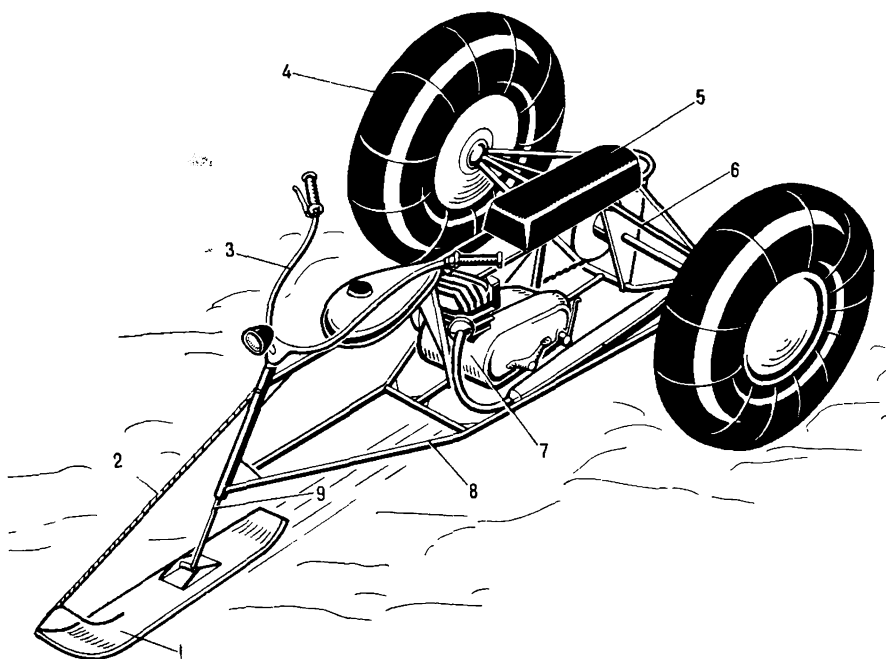
Рис. 82. Снегоход;
