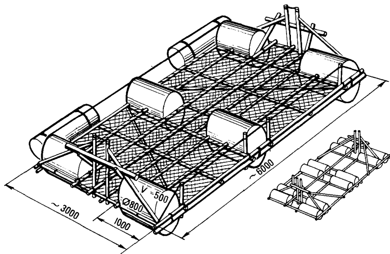
Рис. 134. Ячеистые плоты с одинарными (слева) и двойными (справа) гондолами конструкции А. Фомина
