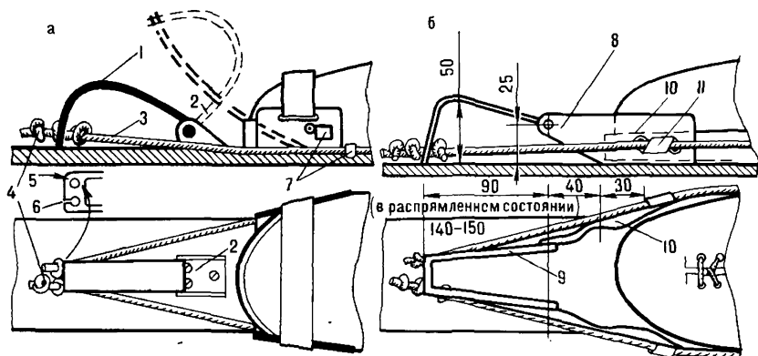
Рис. 61. Лыжные крепления с натяжным устройством:
