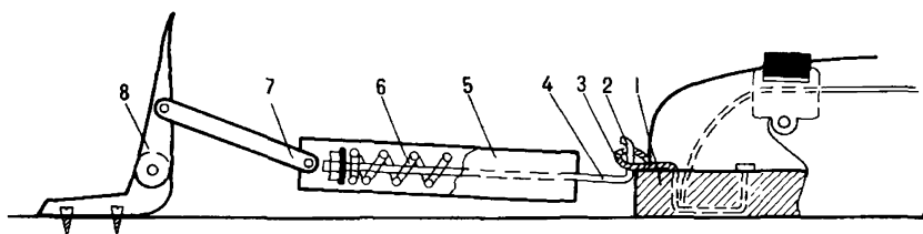
Рис. 62. Бестросиковые крепления с пружиной натяжения типа "безмен"
