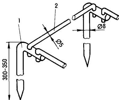
Рис. 30. Разборный таганок
