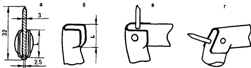
Рис. 88. Стыковка шпангоутов
