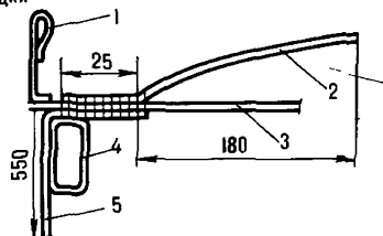
Рис.111. Вшивание строп для крепления спасконца:
