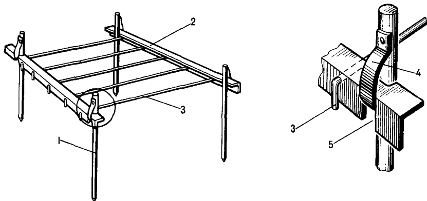
Рис.32.Разборный таганок
