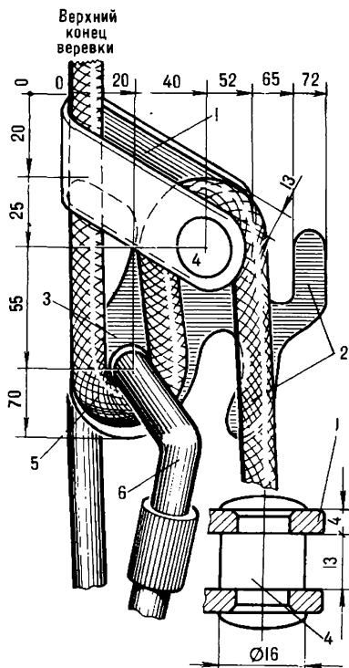
Рис. 223. Фрикционное устройство
