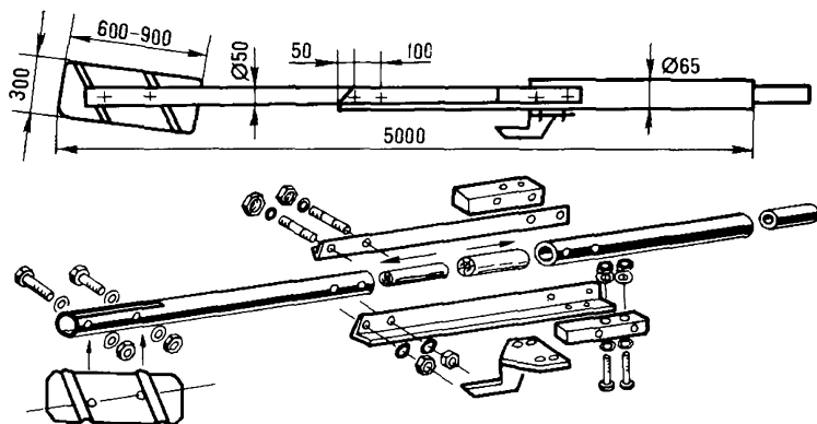
Рис.138. Металлическая гребль из труб
