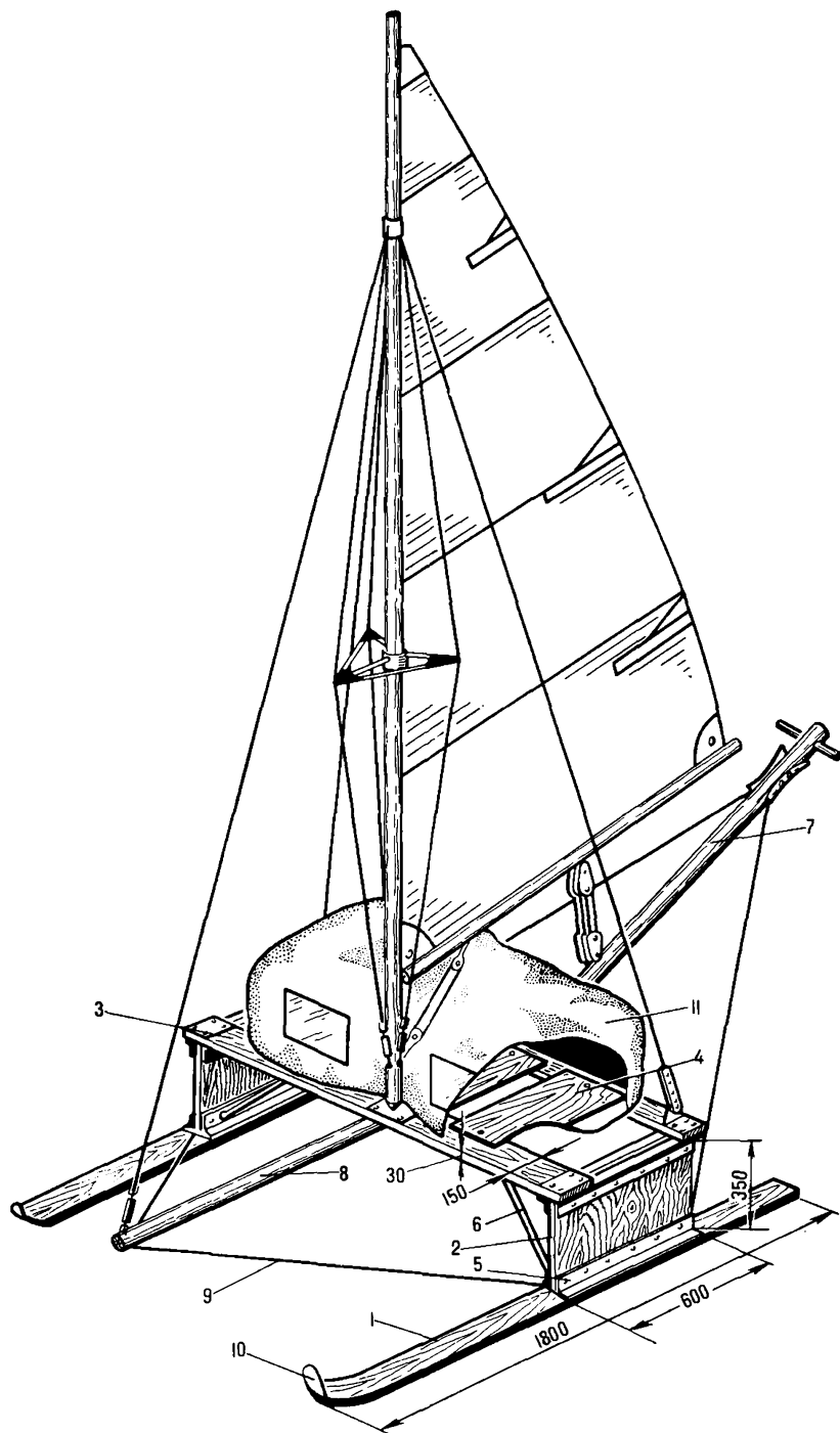
Рис. 80. Парусные карты
