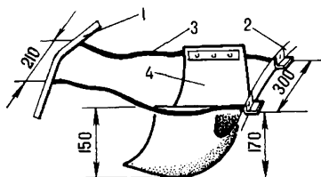
Рис.100. Установка трубчатых упоров: 1—шпангоут; 2—шпангоут; 3—трубчатые упоры; 4—банка
