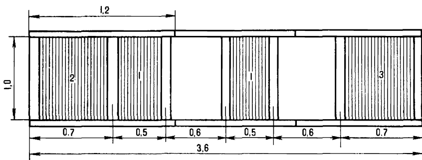
Рис.116, Основные размеры каркаса и вариант разнеса поперечин (размеры в м): 1-места посадки членов экипажа; 2-кормовой; 3-носовой багажники
