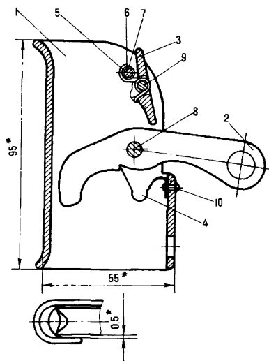
Рис 197. Кулачковый зажим конструкции Абалакова : 1—корпус; 2—рычаг, 3—зашелка; 4 и 5—пружины; 6, 8, 9—оси, расклепать, обеспечить свободный поворот рычага (суммарный зазор 1 мм); не указанные предельные отклонения размеров: по СМ; покрытие Ан Окс хр; 7—штулка, 10—заклепка 2×6—711 ГОСТ 10299—68; размеры для справок. Острые кромки скруглить до R=0,5 мм
