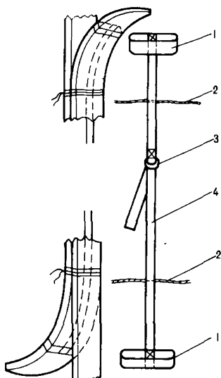
Рис. 45. Ременная система для связывания лыж. При использовании их в качестве опоры палатки: 1 - кольца из капроновой тесьмы диаметром меньше широкой части носка лыжи; 2 - тесьма для связывания лыж; 3 - пряжка из двух колец; 4 - капроновый фал
