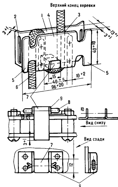
Рис. 224. Пряжка-фрикцион
