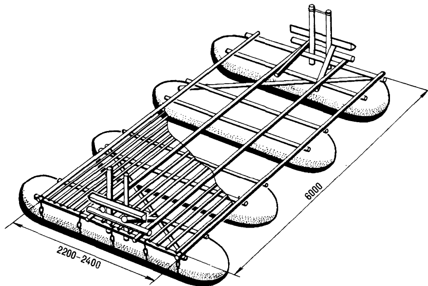
Рис. 133. Понтонный плот
