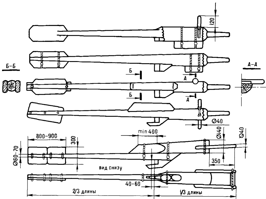
Рис.137. Деревянные гребни и варианты их узлов
