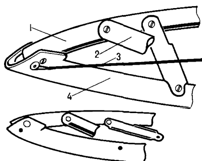
Рис. 94.Стыковка штевневых окончаний с откидным пиллерсом :
