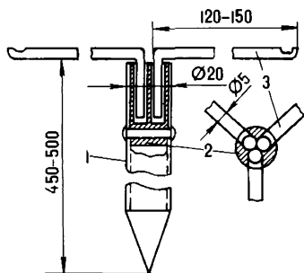
Рис. 29. Костровая вешалка
