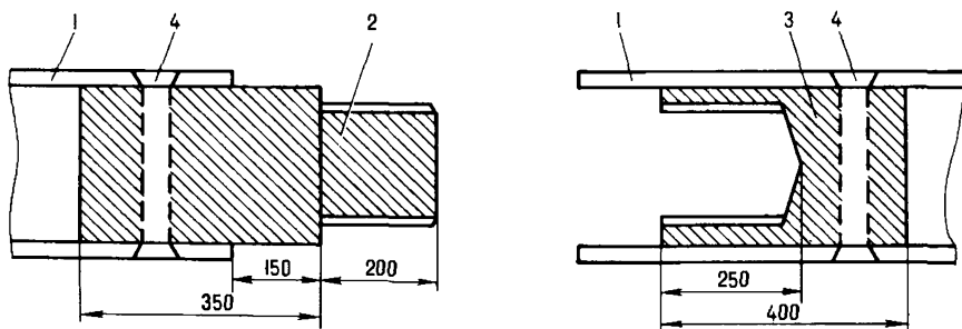
Рис. 76. Лавинный зонд из лыжных палок:
