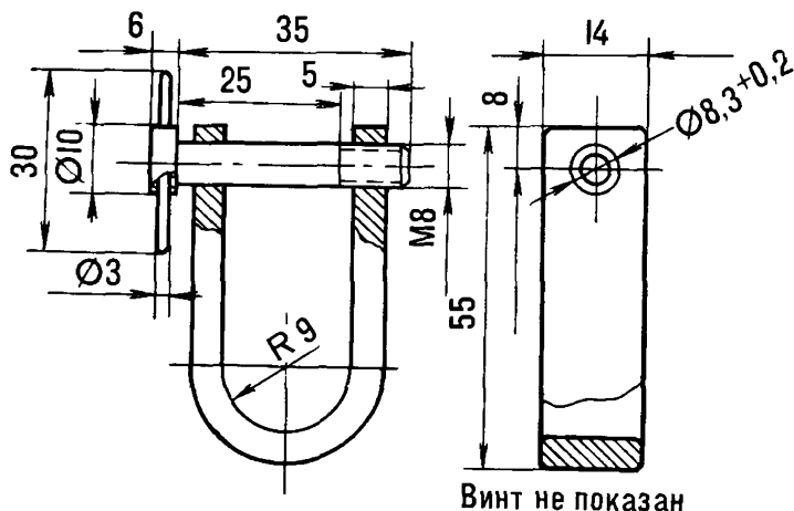
Рис.229.Карабин для навески снаряжения
