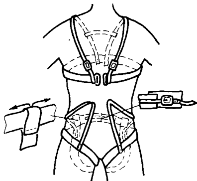
Рис.195. Комбинация грудной обвязки и беседки
