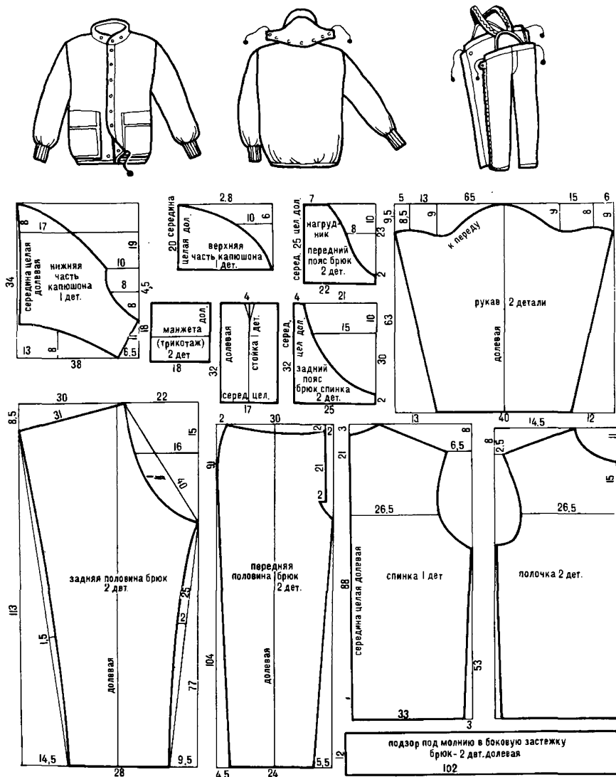
Рис. 23. Пуховый костюм (размеры в см)
