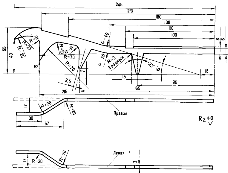
Рис.182 Кошка конструкции Муравьева. Боковины передка Материал: сталь 4Х13. На одну пару кошек идет две пары боковин передков. Острые кромки притупить.
