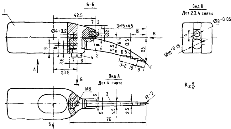
Рис. 166. Молоток альпинистский: 1—головка (ОСТ62-99-78); 2—вставка из твердого сплава ВК-8, ВК-10 (зачеканивается в головку молотка) 3—клюв (сталь 30ХГСА, твердость клюва HRC 40-45); 4—винт установочный М6×0.75 Неуказанные предельные размеры: отверстий—по А 7, валов—по В 7, остальных по-СМ 7. Неуказанные радиусы острых кромок—0.5 мм; на поверхности Г острые кромки сохранить
