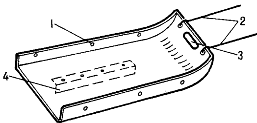
Рис. 67. Волокуша для рюкзака из дюралевого листа
