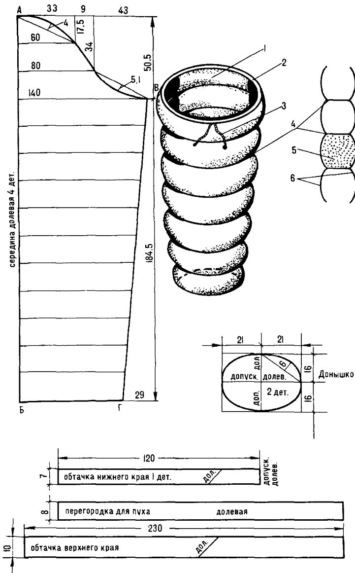
Рис. 9. Спальный мешок "Кокон" (размеры в см.).
