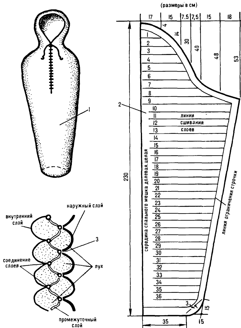
Рис. 8. Индивидуальный спальня мешок типа "Футлар":
