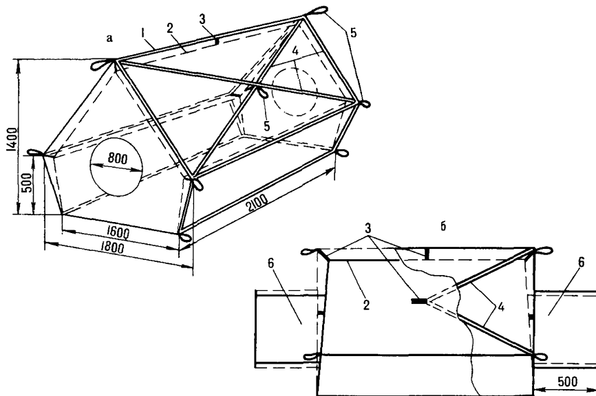
Рис. 3. Двухслойная палатка типа "Памирка":
