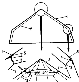
Рис. 44. Крепление второго слоя к наружному слою палатки: 1 - наружный слой палатки; 2 - внутренний слой; 3 - резинка или тесьма; 4 - крючок; 5 - петли из тесьмы
