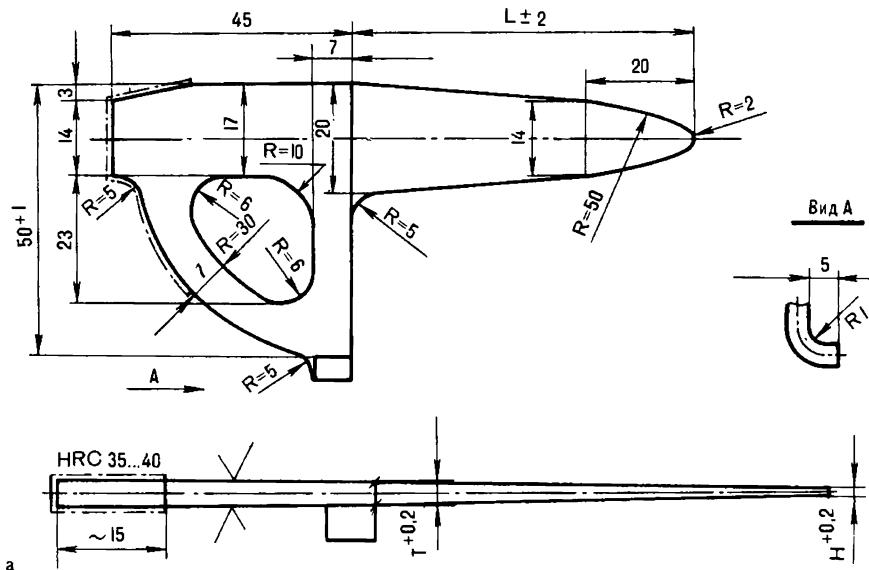
Рис.153. Вертикальный(а) и горизонтальный(б) стальные крючья
