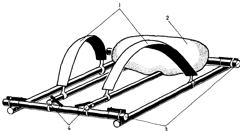
Рис. 124. Место для гребца: 1 — упоры из дюралевых пластин или капроновых ремней; 2 — мешок с личными вещами (возвышается над баллоном на 20-25 см); 3 — поперечины; 4 — дюралевые трубки диаметром 20 мм
