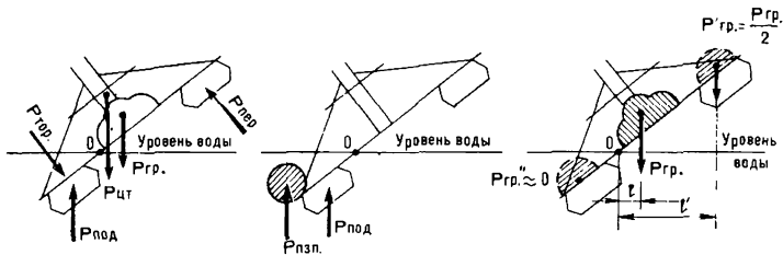
Рис.128. Действие сил, влияющих на остойчивость плота
